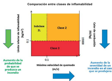
Figura 1.13: Comparación entre clases de inflamabilidad.
